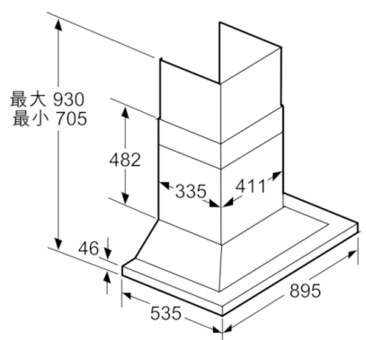
尺寸 (毫米)
