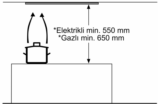
* Ocak ızgarasının üst kenarından itibaren Ölçüler mm cinsindendir
