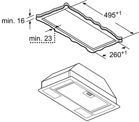
Ölçüler mm cinsindendir
