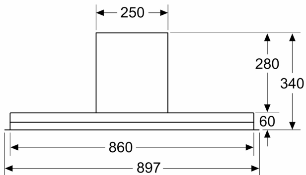
Mått i mm Frontvy
