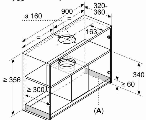
Mått i mm Inbyggnadsexempel
