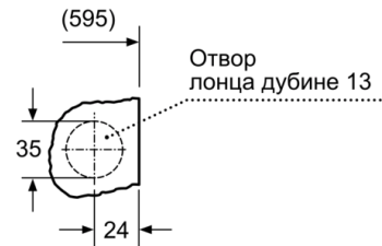
Детаљ Z
