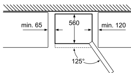
Dimenzije v mm
