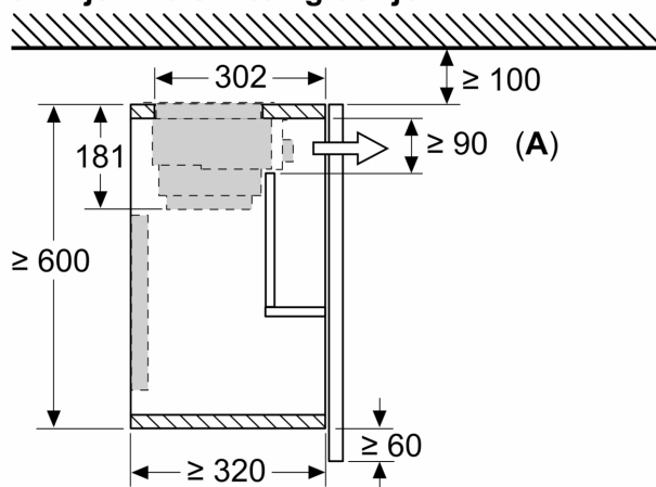
Dimenzije v mm Montaža vgradne izvlečne nape s kompletom za recirkulacijo zraka in okvirjem za skrito vgradnjo
