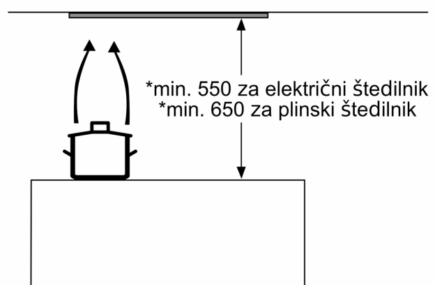
* od zgornjega roba nosilca za posodo Dimenzije v mm
