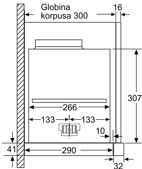
Dimenzije v mm
