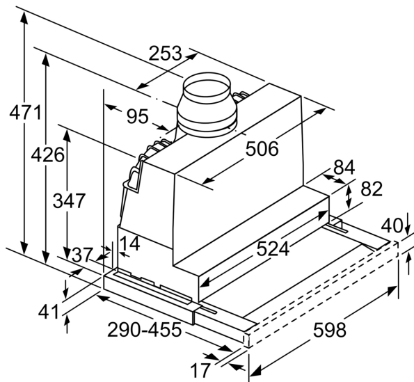
Prilagoditev globine izvleka filtra je mogoča do 29 mm Dimenzije v mm
