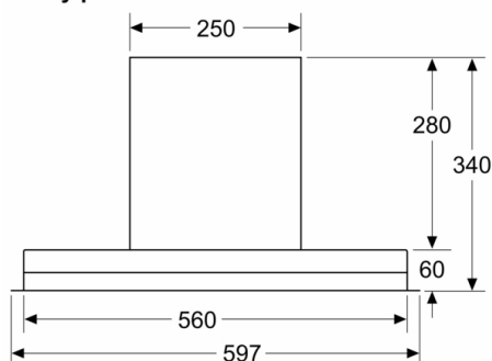
rozmery v mm Čelný pohľad
