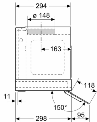
rozmery v mm pohľad z boku
