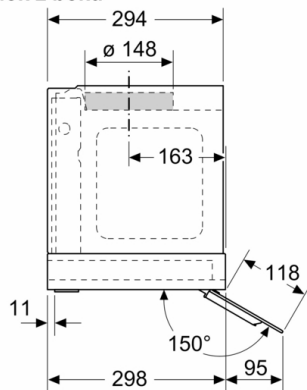
wymiary w mm widok z boku
