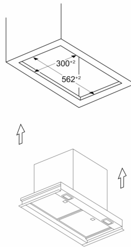
Afmeting in mm Installatievoorbeeld in meubeluitsparing
