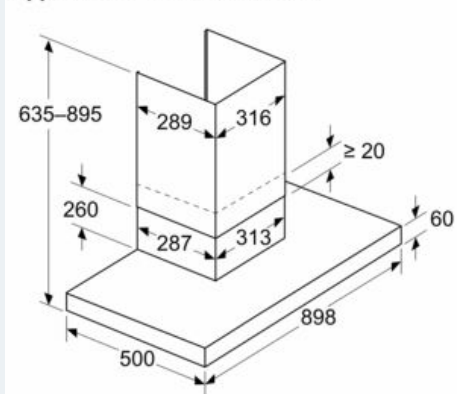
Afmeting in mm Apparaat in luchtvoermodus
