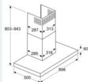
Recirculatiemodus met recirculatieset (de recirculatieset is uitsluitend beschikbaar als afzonderlijk accessoire)
