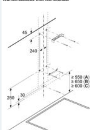
Afmeting in mm Wandinstallatie met luchtkanaal
