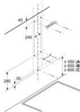
Afmeting in mm Wandpaneeldiepte
