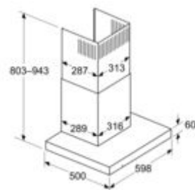
Afmeting in mm Recirculatieperspectief
