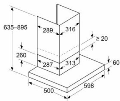
Afmeting in mm Apparaat in luchtafvoermodus
