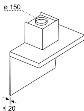
Afmeting in mm Wandpaneeldiepte
