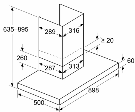
Afmeting in mm Apparaat in luchttafvoermodus
