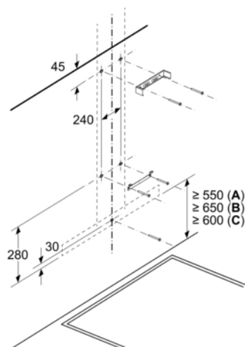
Afmeting in mm Recirculatieperspectief
