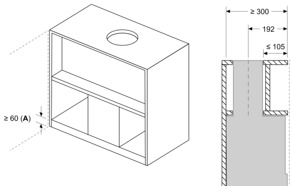
Afmeting in mm Installatievoorbeeld met kruidenrek
