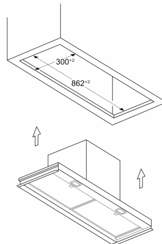
Afmeting in mm Installatievoorbeeld in meubeluitsparing
