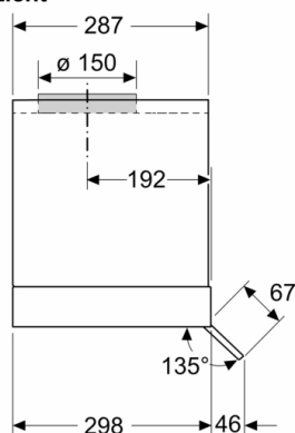
Afmeting in mm Zijaanzicht
