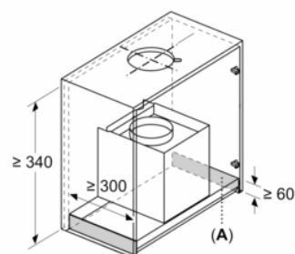
Afmeting in mm Installatievereisten voor vervanging
