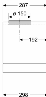
Afmeting in mm Zijaanzicht
