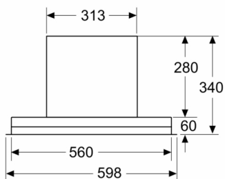
Afmeting in mm Vooraanzicht
