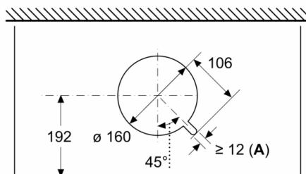
Afmeting in mm Aanzicht van boven
