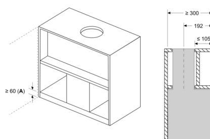
Afmeting in mm Installatievoorbeeld met kruidenrek
