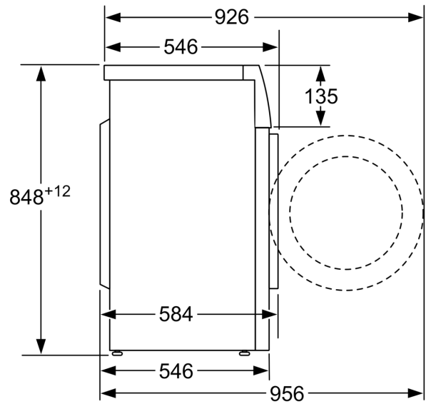
Izmēri (mm)
