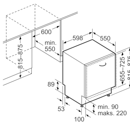
Izmēri (mm)
