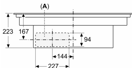
Izmēri mm Skats no priekšpusē
