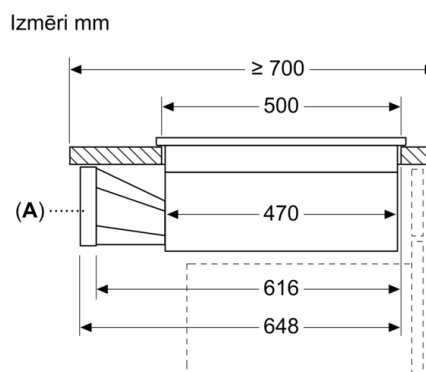
A: Apaļas-plakanas formas adapters
