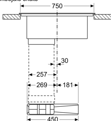
Izmēri (mm) Priekšējais skats
