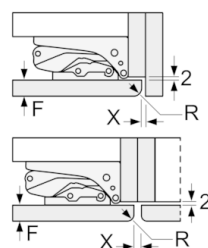
Izmēri mm Plakanā šarnīra spraugas izmēru ieteikums
