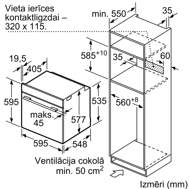
Izmēri (mm)
