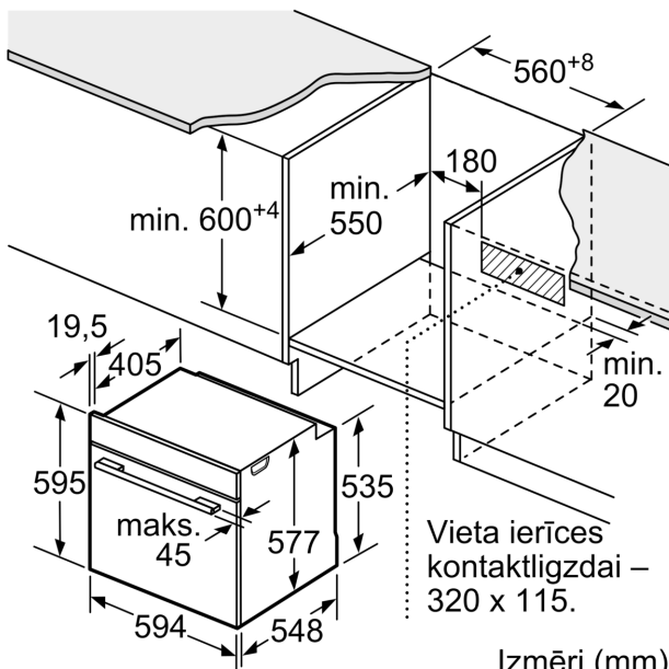
Izmēri (mm)
