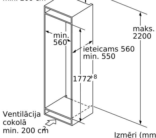
Izmēri (mm)
