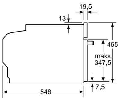
Izmēri (mm)
