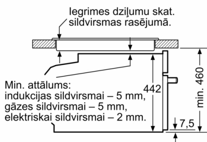
Izmēri (mm)
