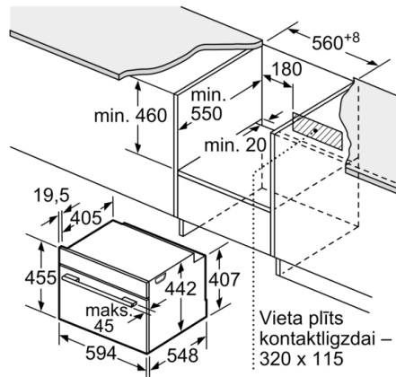
Izmēri (mm)
