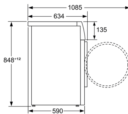
Matmenys, mm
