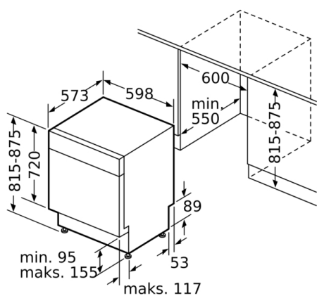
Matmenys, mm
