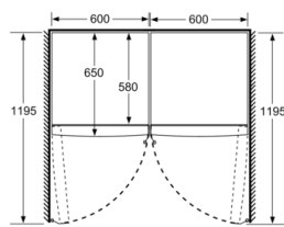
Matmenys, mm
