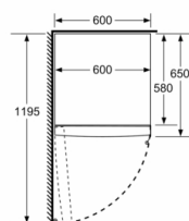
Matmenys, mm
