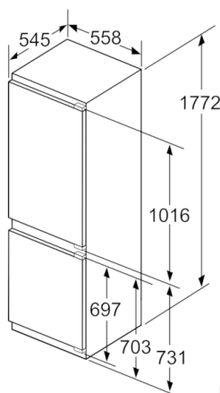
Matmenys, mm
