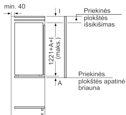
Matmenys, mm
