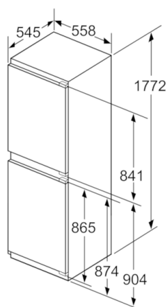
Matmenys, mm
