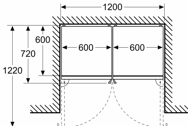
Matmenys, mm
