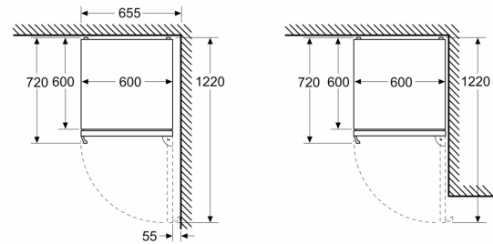
Matmenys, mm
