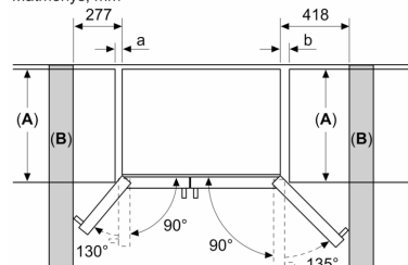
Matmenys, mm
