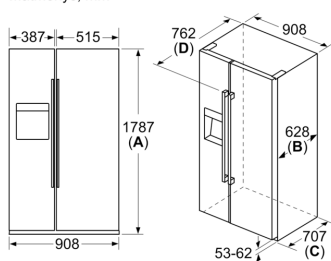
Matmenys, mm
