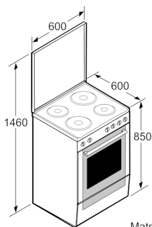
Matmenys, mm
