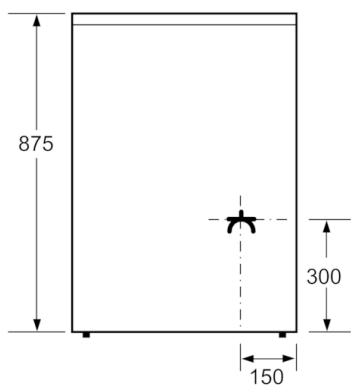
Matmenys, mm
