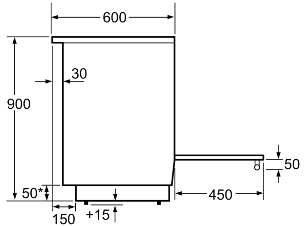
Matmenys, mm
