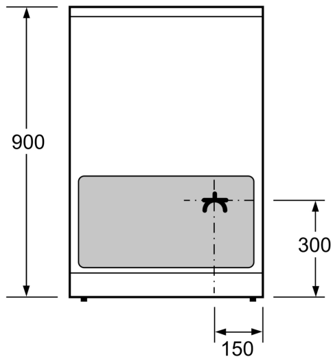
Matmenys, mm
