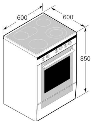
Matmenys, mm
