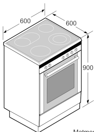
Matmenys, mm
