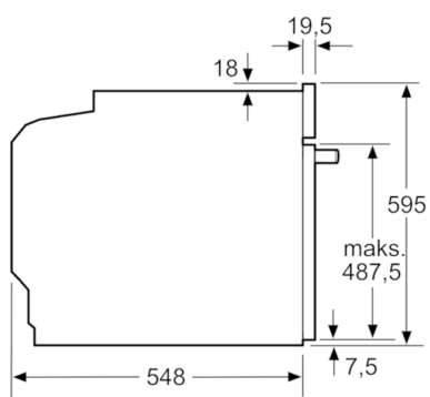
Matmenys, mm
