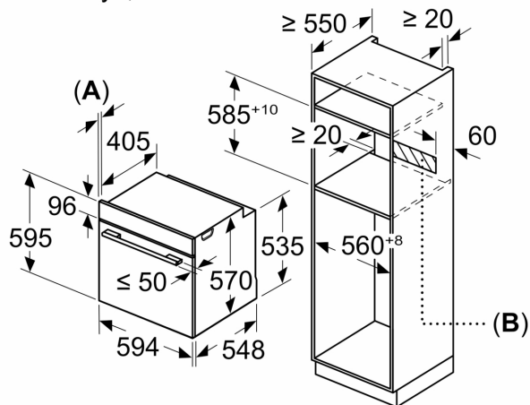
Matmenys, mm
