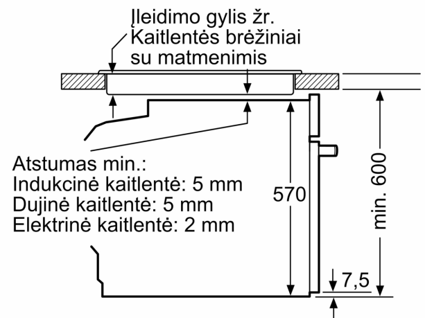
Matmenys, mm
