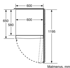
Matmenys, mm
