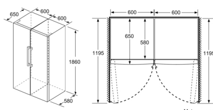
Matmenys, mm
