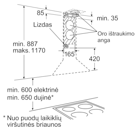
Matmenys mm
