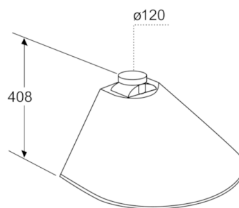
Matmenys mm
