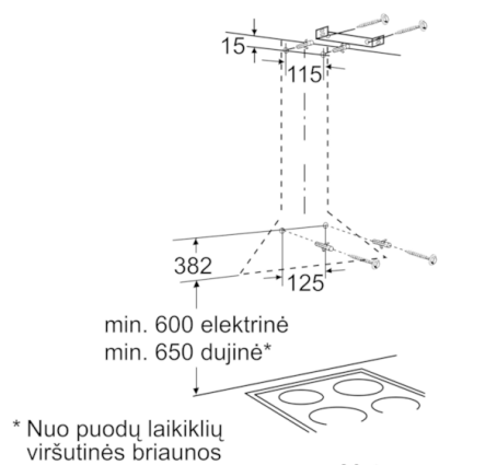
Matmenys mm
