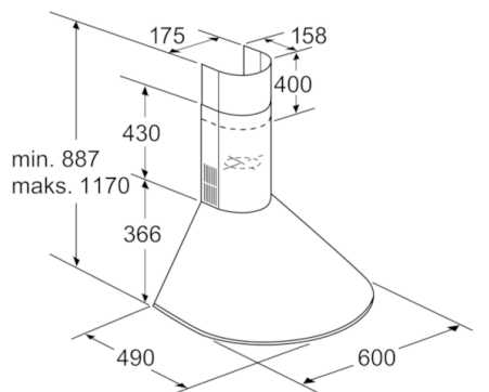
Matmenys mm
