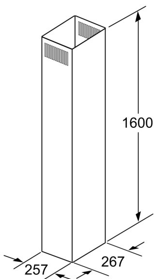
Matmenys, mm
