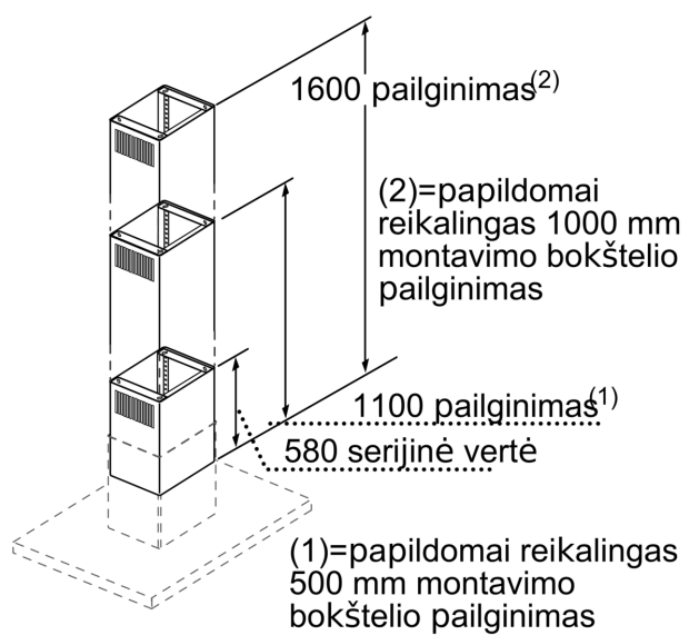
Matmenys mm
