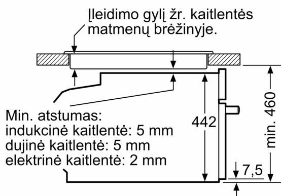
Matmenys, mm
