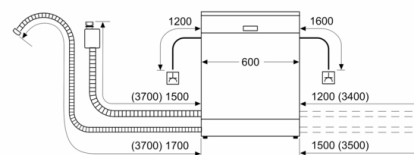
Dimensioni in mm
