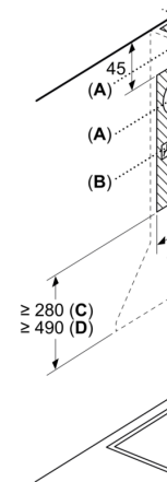
Dimensioni in mm
