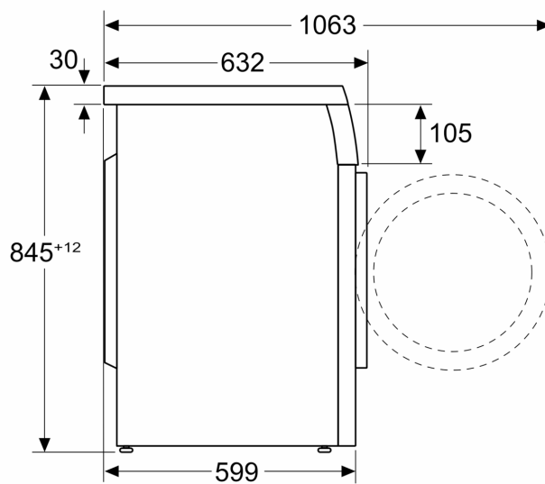
Méreték mm-ben
