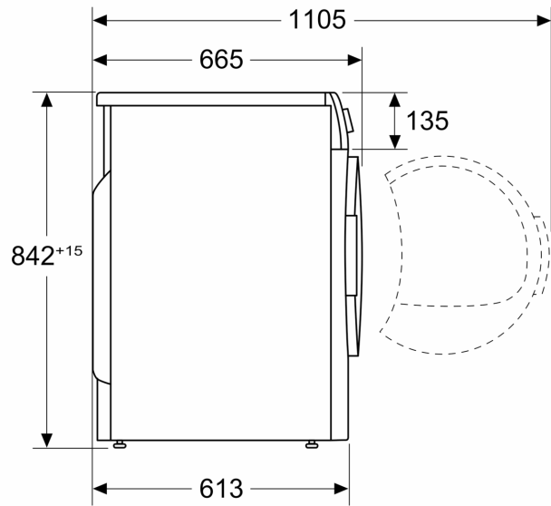
Méretetek mm-ben
