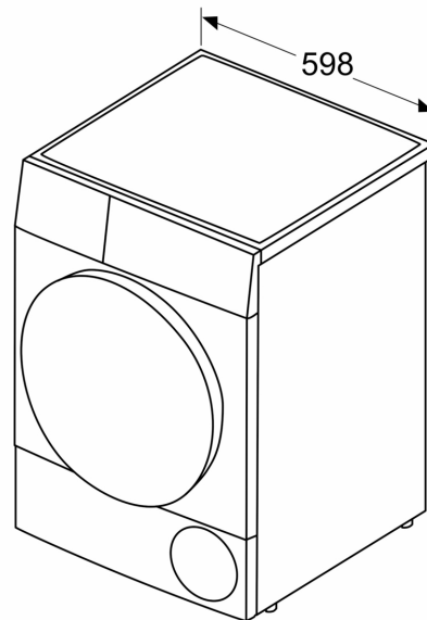
Méretetek mm-ben
