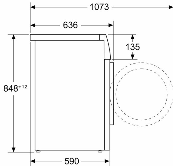
Méreték mm-ben
