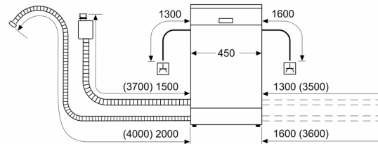
méretek mm-ben
